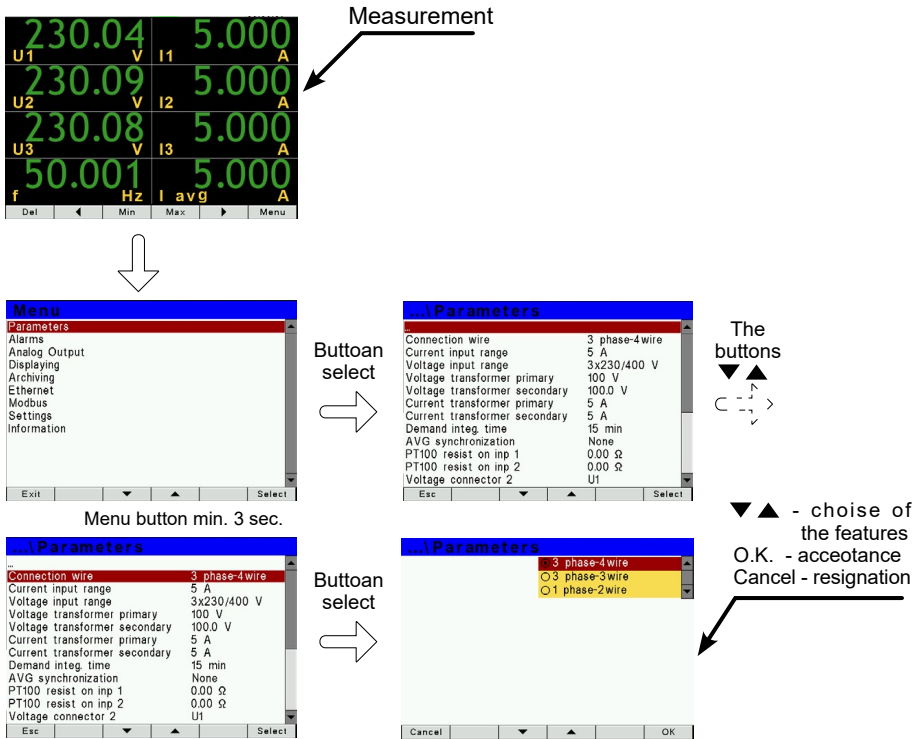
Fig. 23. Screens of Parameters mode
